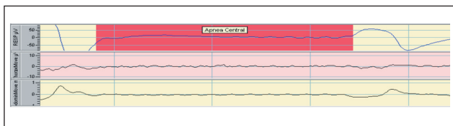
FIG. 14.18 Apneia mista: Apneia com uma primeira fase central e uma segunda fase obstrutiva
