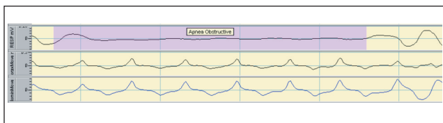
FIG. 14.16 Apneia obstrutiva: Ausência de fluxo nasal mantendo movimentos torácicos e abdominais
